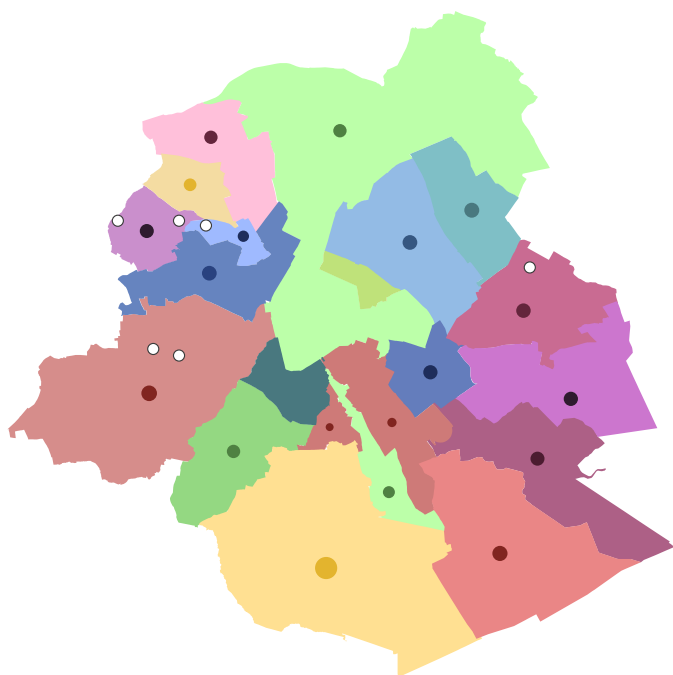
○ LISA-antennes
